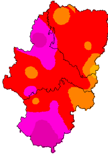
SPI12 (mayo de 2020)
