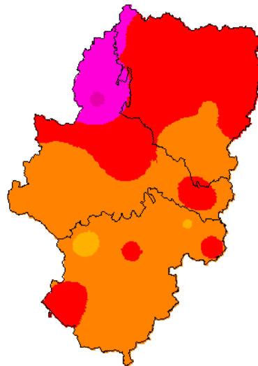
SPI3 (mayo de 2020)
