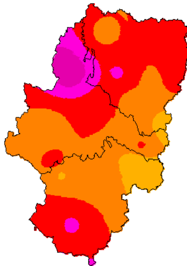
SPIAÑOAGRICOLA(9 MESES) (mayo de 2020)
