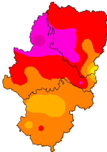
SPI24 (mayo de 2020)
