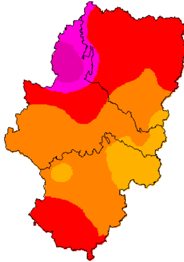
SPI6 (mayo de 2020)
